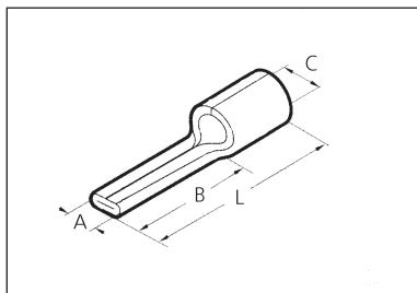
Наконечник силовой "плоская игла" без изоляции Материал - луженая медь
