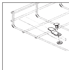
Крепеж лотка к основанию кронштейна*
