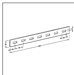
Соединитель боковой регулируемой длины Длина - 3м
