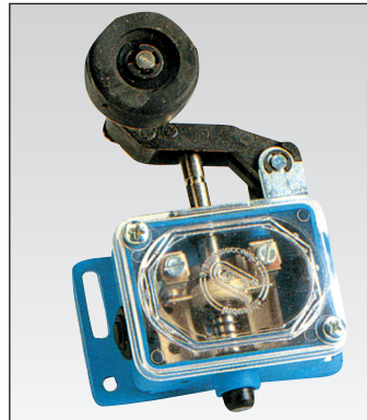
Концевой выключатель Привод - рычаг с роликом Ø 35 мм
