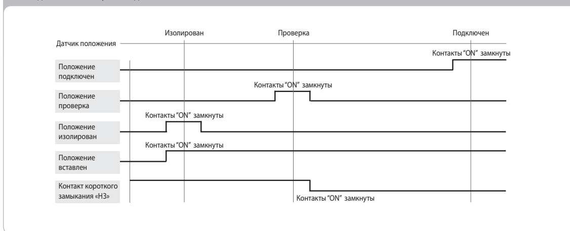
Последовательность работы датчиков положения
